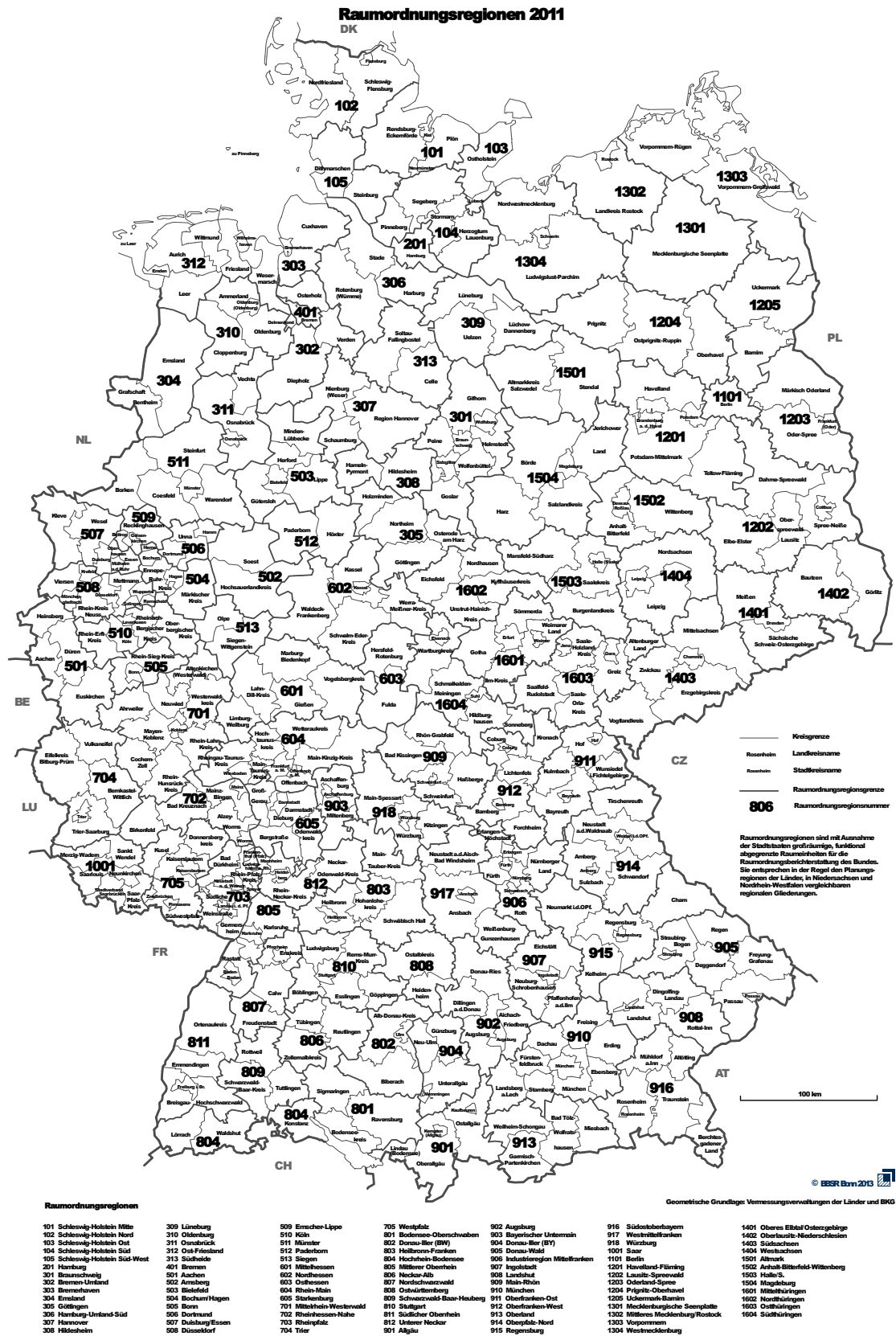
Figure B1: LOCAL LABOR MARKETS, 96 RAUMORDNUNGSREGIONEN [ROR]
