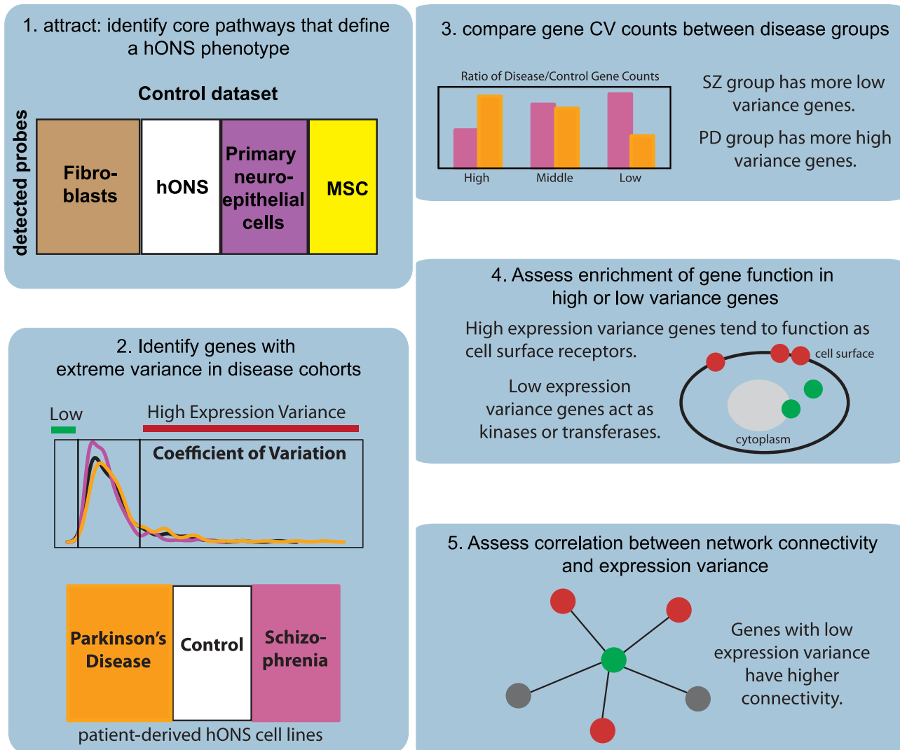
Figure 1. Overview of analysis pipeline. doi:10.1371/journal.pgen.1002207.g001
