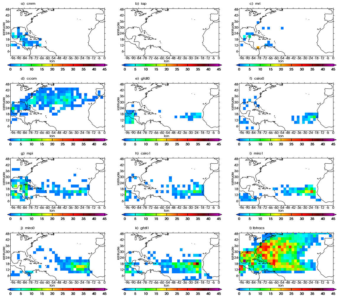
Figure 2: Density of TCs detected over JAS 1980-1998 over the North Atlantic basin : a) cnrm, b) iap, c) mri, d) ccam, e) gfdl0, f) csiro0, g) mpi, h) csiro1, i) miro1, j) miro0, k) gfdl1 and l) Ibracs.
