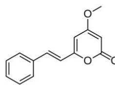
DESMETHOXYANGONIN
